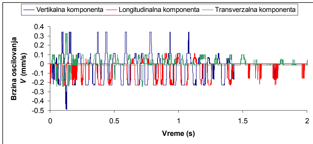
Slika 4-3. Velosigrani vertikalne, longitudinalne i transverzalne komponente brzine oscilovanja izmerene pri miniranju 18.08.2010. u 14:21 h
