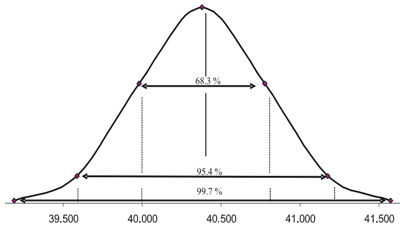
Slika 2-17. Normalna raspodela vremena usporenja NONEL konektora sa nominalnim vremenom usporenja od 42 ms
