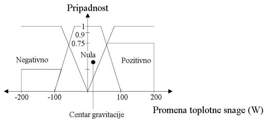
Slika 5-8. Metode defazifikacije [108]
