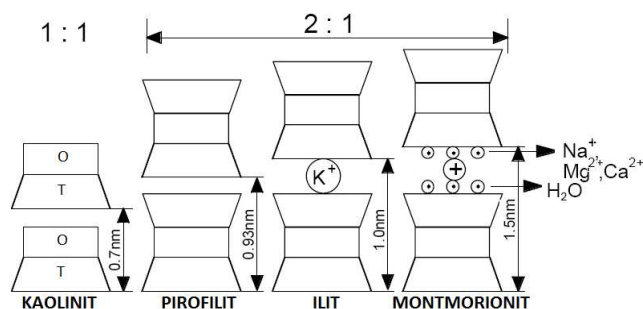
Slika 1. Strukturni prikaz za 1:1 i 2:1 slojevitost strukturu, O i T obeležja se odnose na oktaedarski i tetraedarski sloj ( http://ramaseshan.com/Images/phillosilicates.jpg )
