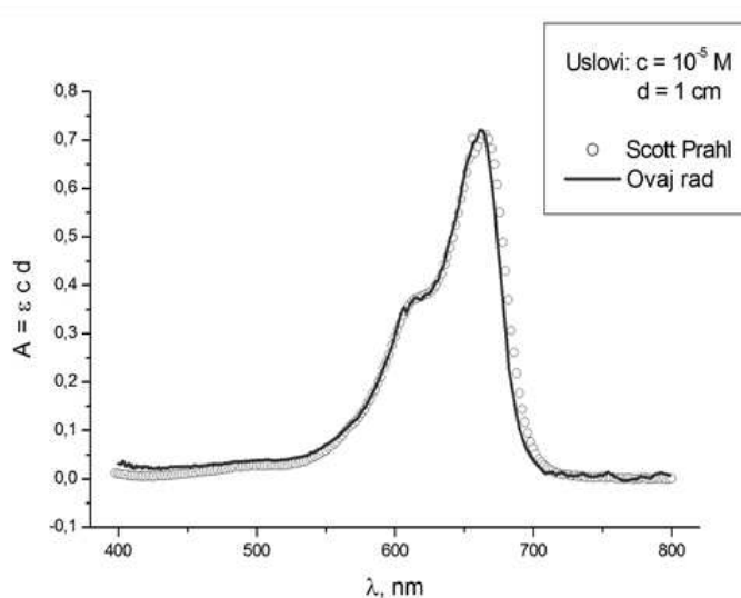
Slika 19. Izračunati i izmereni spektri MB (Milošević, 2011)
