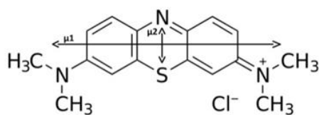
Slika 8. Šematski prikaz strukture molekula metilen plavog sa glavnim ( \mu_1 ) i sekundarnim ( \mu_2 ) dipolnim elektronskim prelazom (Milošević et al. , 2013)
