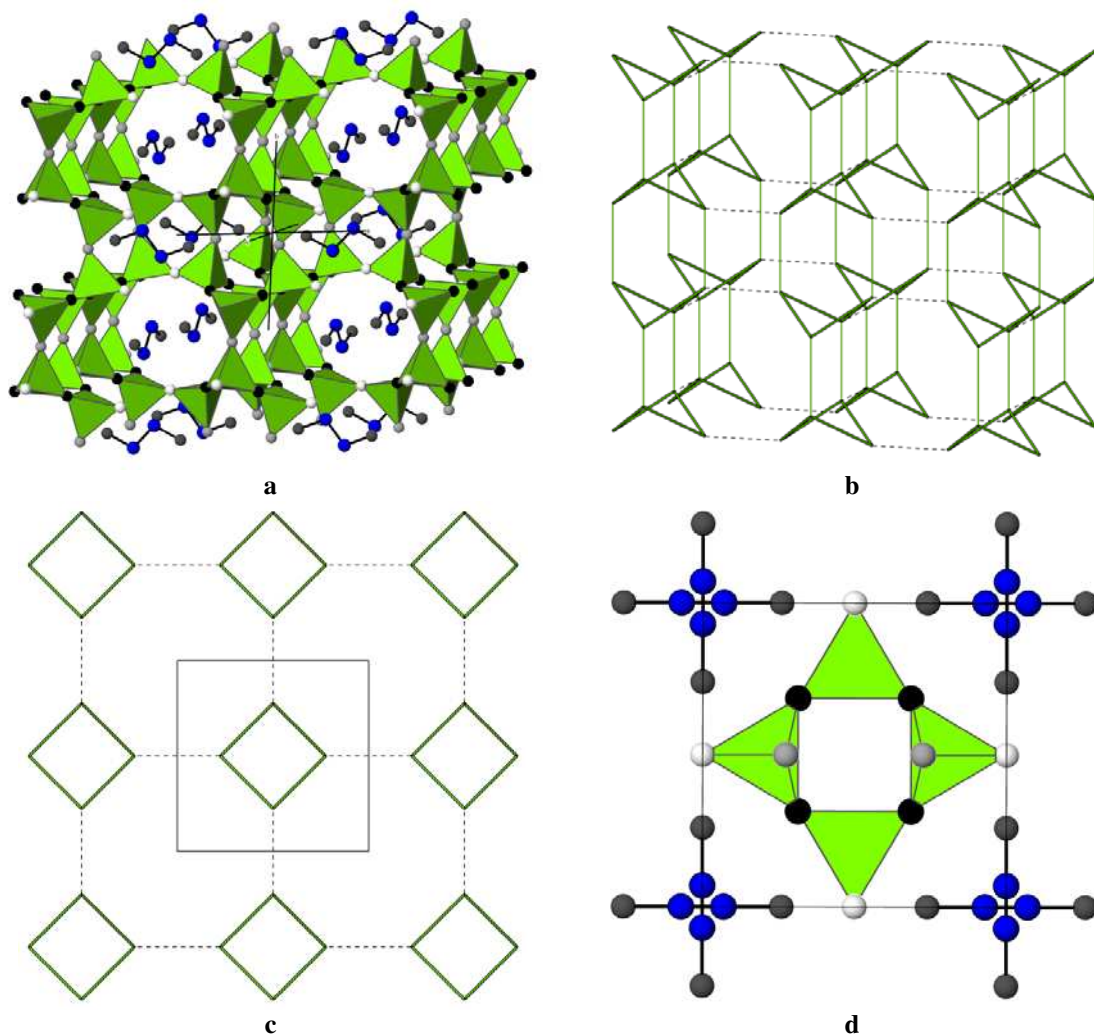
Slika 17. Tetragonalni aristotip strukture zeolita sa DFT-topologijom: a) 3D mreža tetraedara vezanih preko rogljeva i 8M kanali ispunjeni H_2en^{2+} -kationima gledano približno duž [100] . Atomi vodonika su izostavljeni zbog preglednosti, b) veza bhs lanaca izgrađenih od 4M tetraedarskih prstenova povezanih u 3D mrežu gledano približno duž [100] , c) dvodimenzionalna 4.8^2 mreža normalna na [001] sa 4M i 8M tetraedarskim prstenovima, centralni kvadrat (tanka puna linija) predstavlja jediničnu ćeliju, d) pravilni SiO_4 tetraedri povezani u 4M tetraedarske prstenove sa H_2en^{2+} duž [100] i [010] u jediničnoj ćeliji gledano duž [001] . Atomi kiseonika O1 su crni, O2 svetlo sivi, a O3 beli. Atomi azota N1, iz H_2en^{2+} , su tamno sivi, a ugljenika C1 su plavi.
