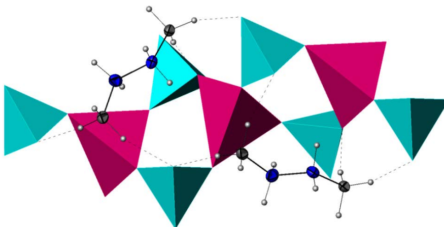
Slika 29. Poliedarski prikaz dela strukture ZnP2 sa lancima ZnP_2O_8^{4-} izgrađenim od tetraedara ZnO_4 (ružičasti) i PO_4 (tirkizni) koji su povezani preko zajedničkih rogljeva. Lanci su vodoničnim vezama povezani sa H_2en^{2+} -katjonima. Tamnoplavi elipsoidi predstavljaju C, a tamnosivi N atome. Termalni elipsoidi nacrtani su sa verovatnoćom od 50 %, a sfere H atoma proizvoljnog su radijusa.
