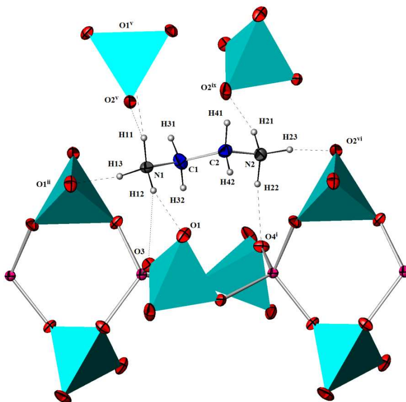
Slika 31. Deo strukture ZnP2 koji prikazuje mrežu vodoničnih veza (isprekidane linije) između NH 3 -grupa iz H 2 en 2+ -katjona i atoma kiseonika iz lanca ZnP 2 O 8 4- . Tačkaste linije predstavljaju manje verovatne vodonične veze. [Simetrijski kodovi: (i) -x+3/2, -y+1/2, z ; (ii) x, -y+1/2, z-1/2 ; (v) -x+2, y-1/2, -z+1/2 ; (vi) x, -y+1/2, z+1/2 ; (ix) x, y-1, z .] Zbog preglednosti prikazani su samo tetraedri PO 4 (tirkizni) iz različitih lanaca.
