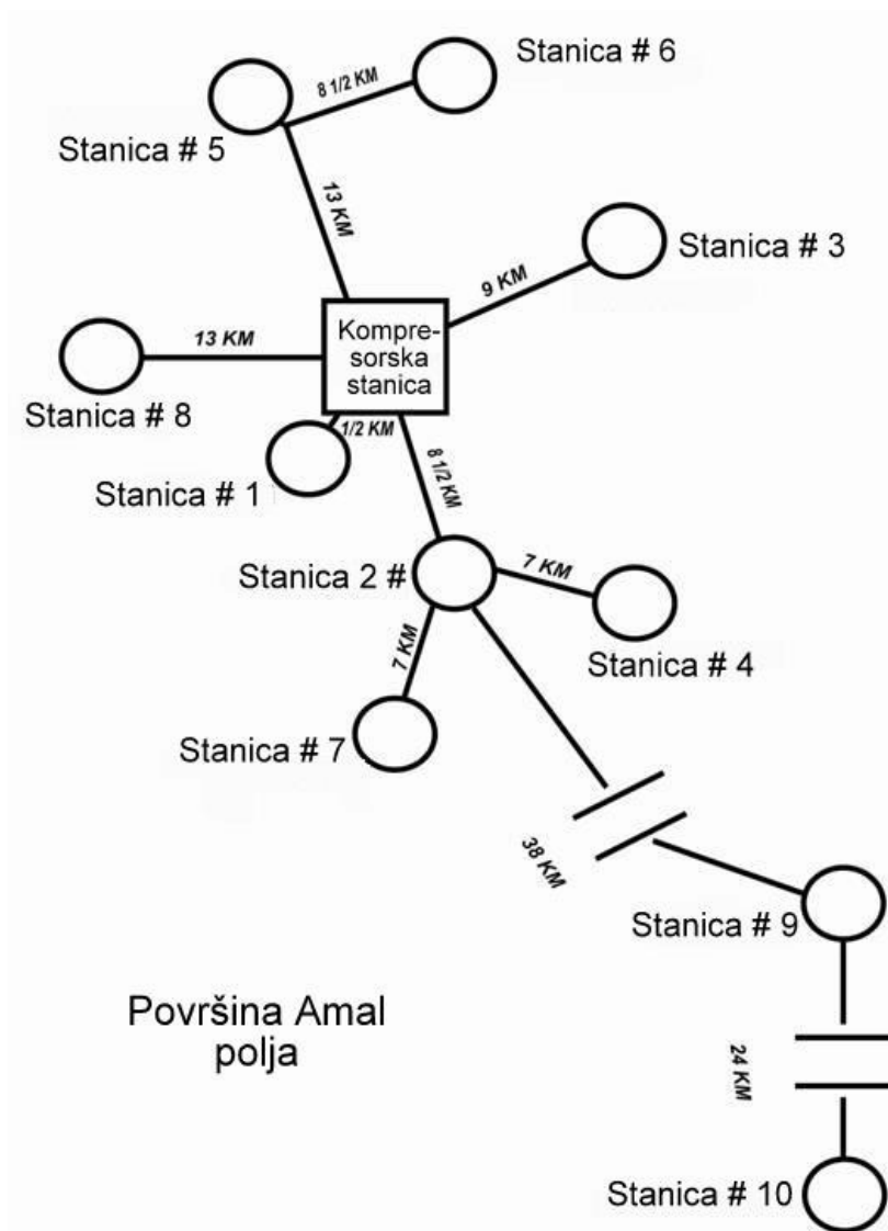
Slika 3.4. Lokacije sabirnih stanica za pripremu nafte i gasa
