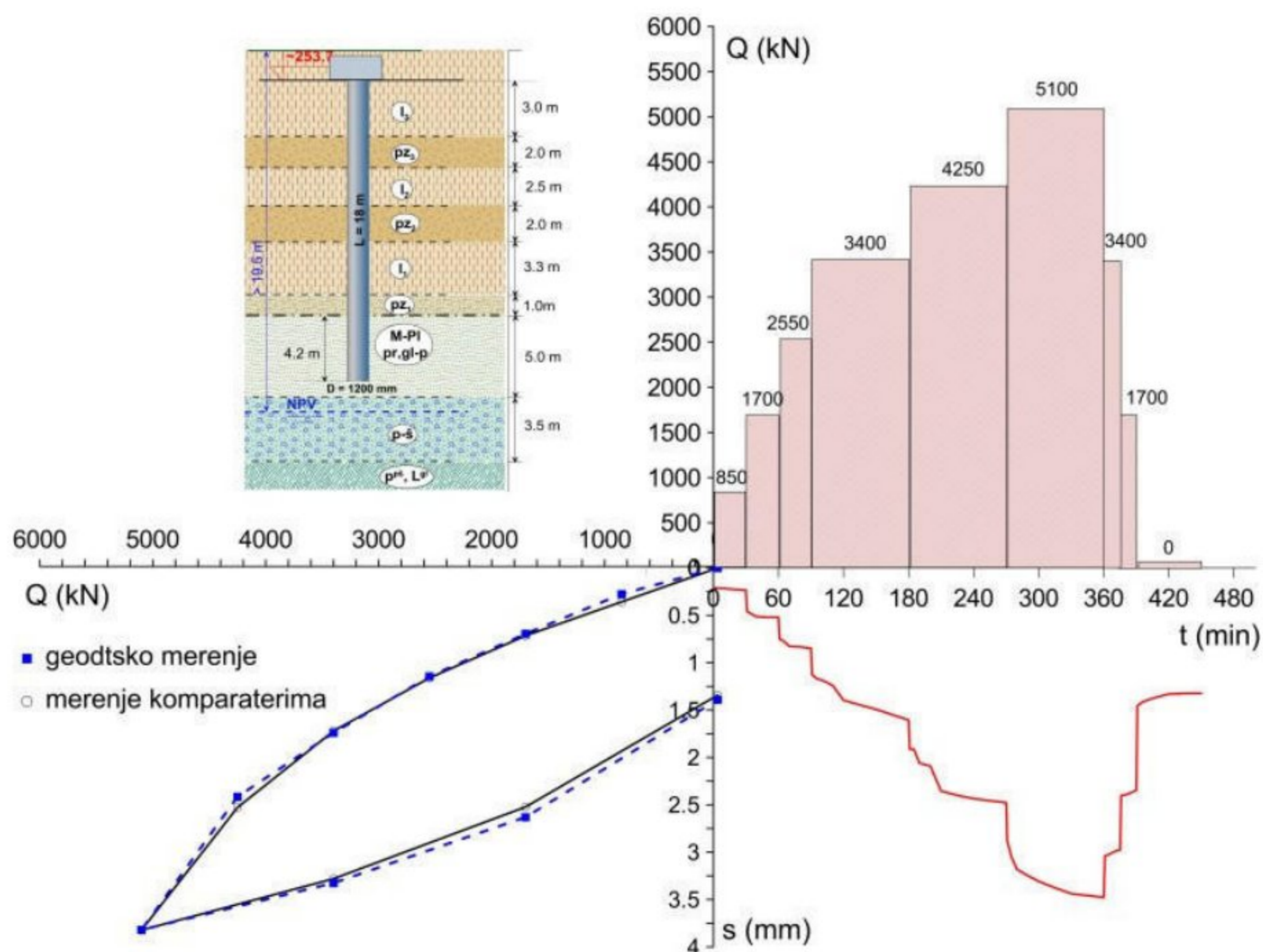
Slika 8. Prikaz rezultata probnog opterećenja šipa
