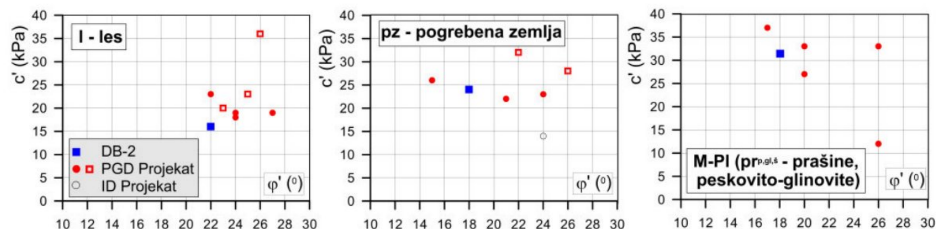
Slika 4. Zbirni prikaz parametara čvrstoće smicanja
