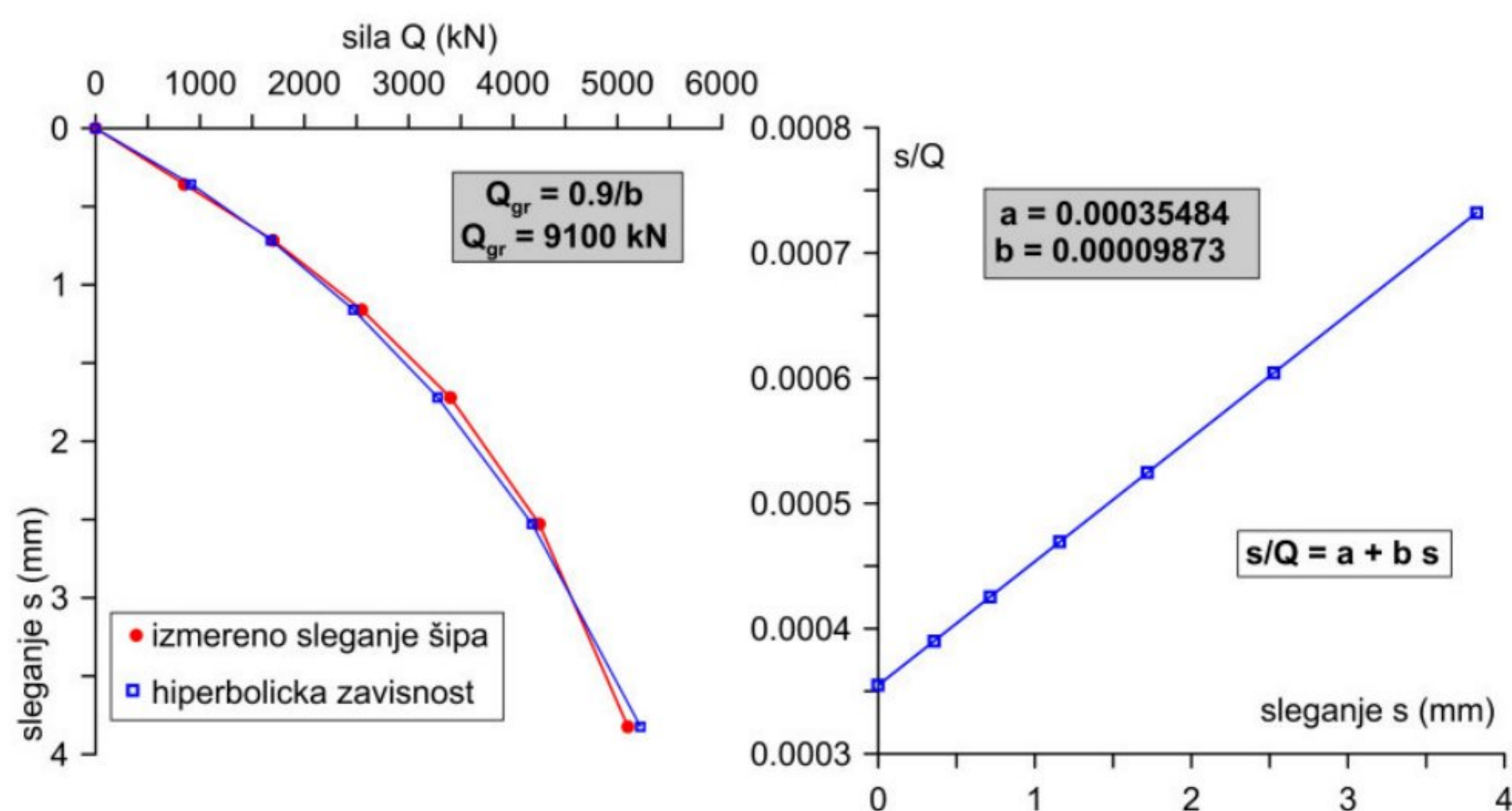
Slika 10. Prikaz definisanja graničnog opterećenja šipa na osnovu hiperboličke zavisnosti
